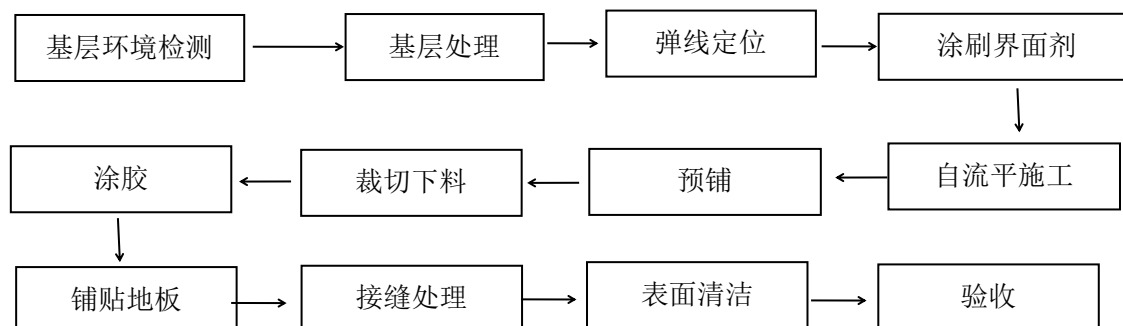
图 14.2.1PVC 地胶安装施工流程示意图
