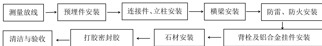
图 22.2.1 石材幕墙安装施工流程示意图
