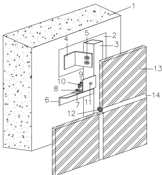
图 22.1.1 铝单板幕墙安装构造示意图
