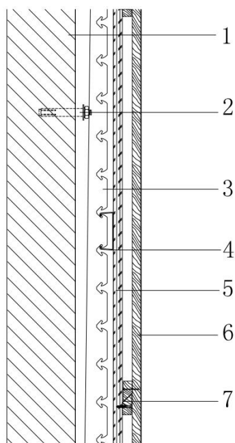
图 10.1.1 木饰面构造示意图
