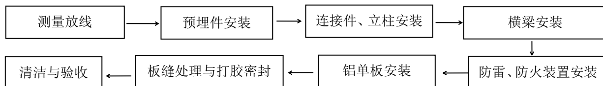
图 21.2.1 铝单板幕墙安装施工流程示意图
