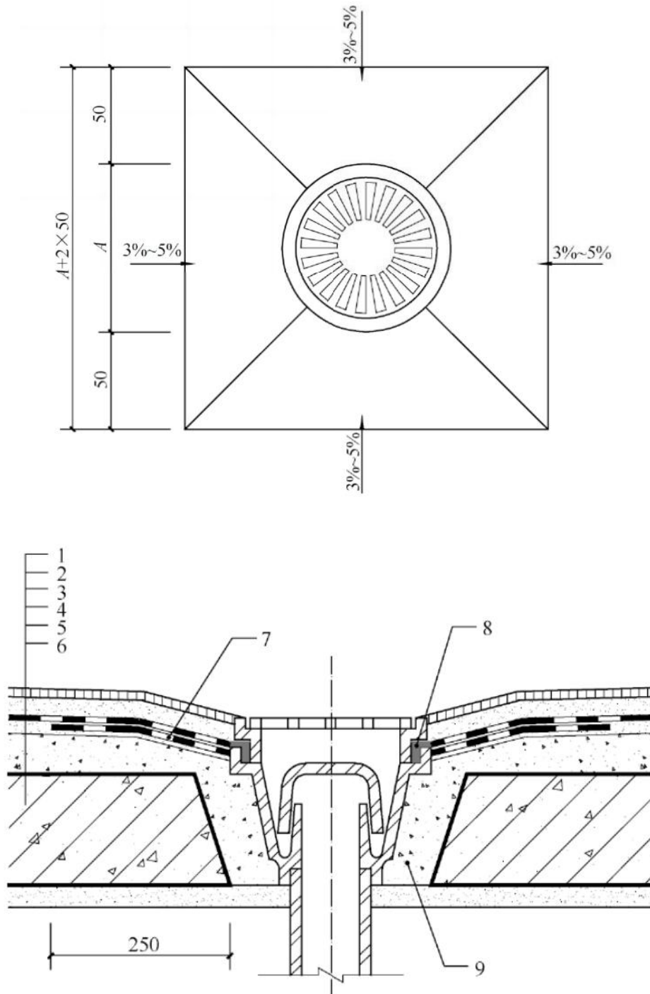
图 19.3.2-3 地漏防水构造
