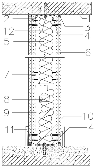
图 7.1.1 轻钢龙骨石膏板隔墙构造示意图
