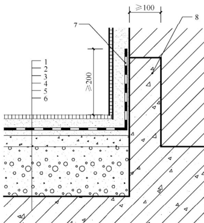
图 19.3.2-5 防潮墙面的底部构造
