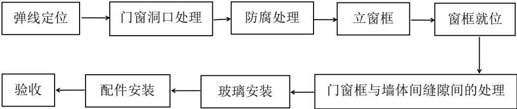
图 15.2.1 断桥铝合金门窗施工流程示意图
