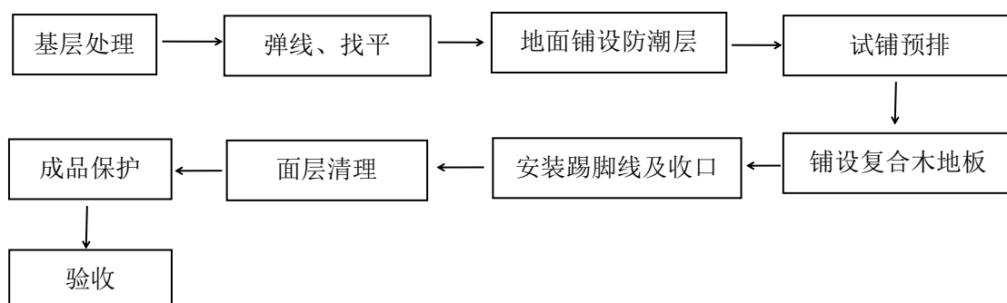
图 13.2.1 复合地板安装施工流程示意图
