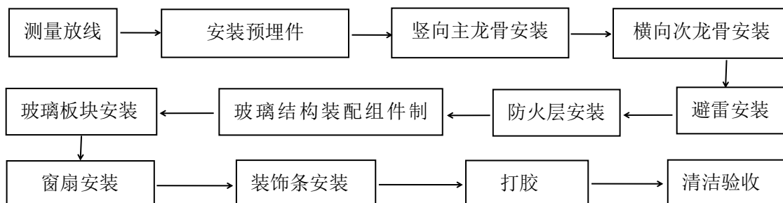
图 20.2.1 玻璃幕墙施工流程示意图
