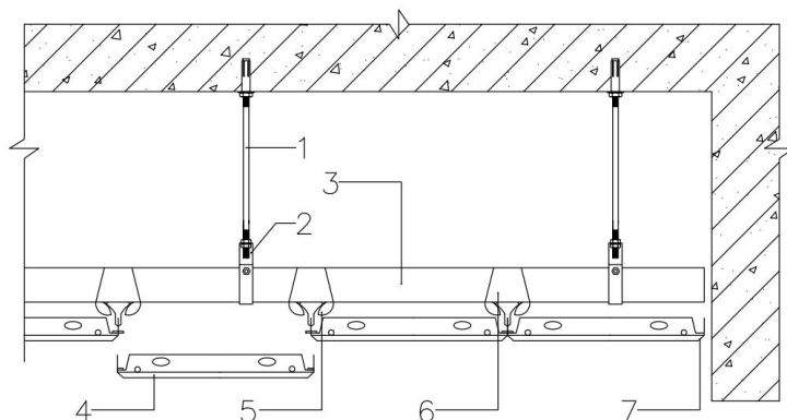
图 6.1.1 铝扣板吊顶构造示意图
