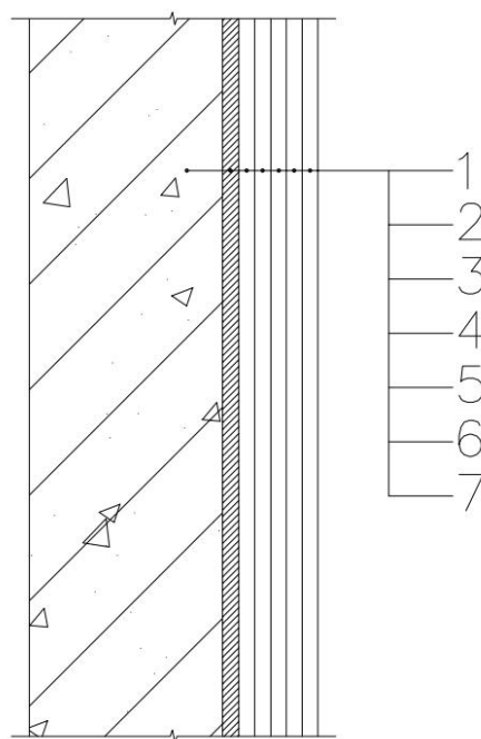
图 11.1.1 涂料构造示意图
