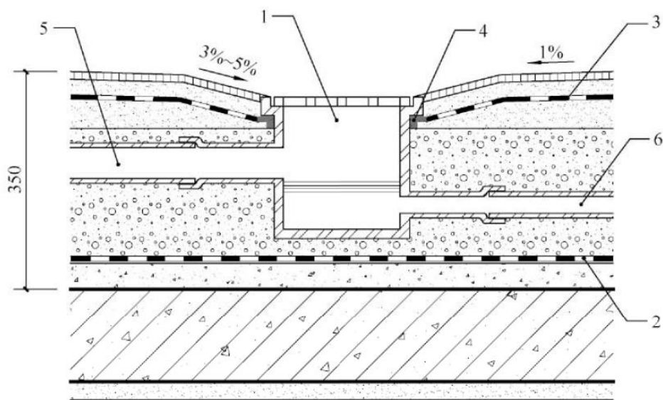
图 19.3.2-5 同层排水时的地漏防水构造
