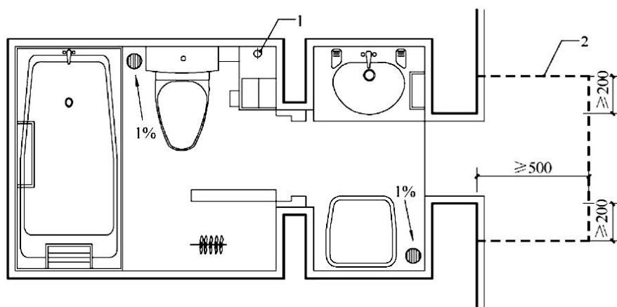
图 19.3.2-1 楼、地面门口处防水层延展示意图
