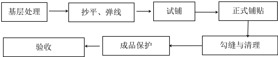
图 12.2.1 地面瓷砖铺贴施工流程示意图
