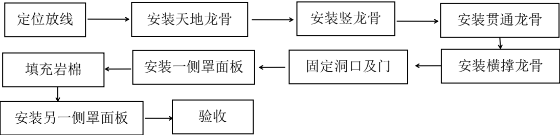
图 7.2.1 轻钢龙骨石膏板隔墙施工流程示意图
