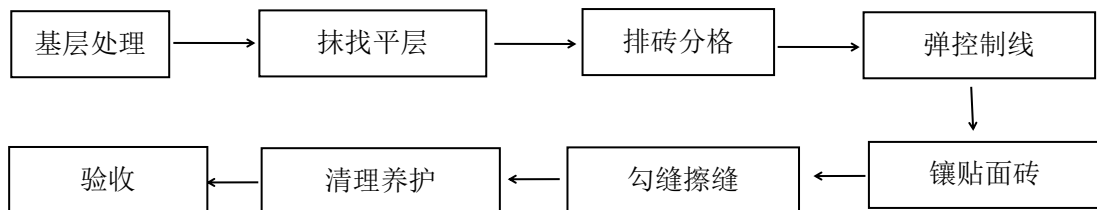
图 8.2.1 饰面砖粘贴施工流程示意图
