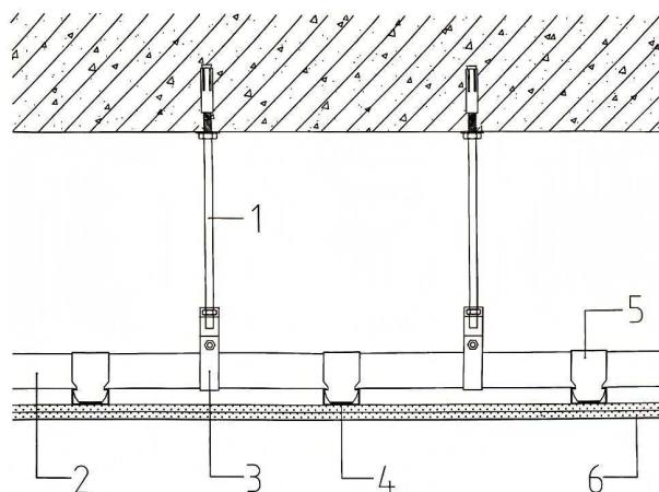
图 5.1.1 轻钢龙骨石膏板吊顶构造示意图
