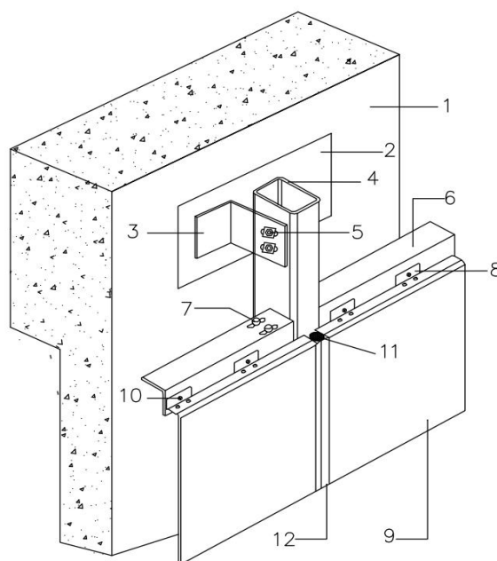
图 21.1.1 铝单板幕墙安装构造示意图
