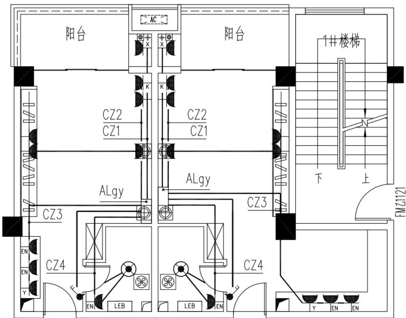
图 17.1.1 电气安装平面示意图
