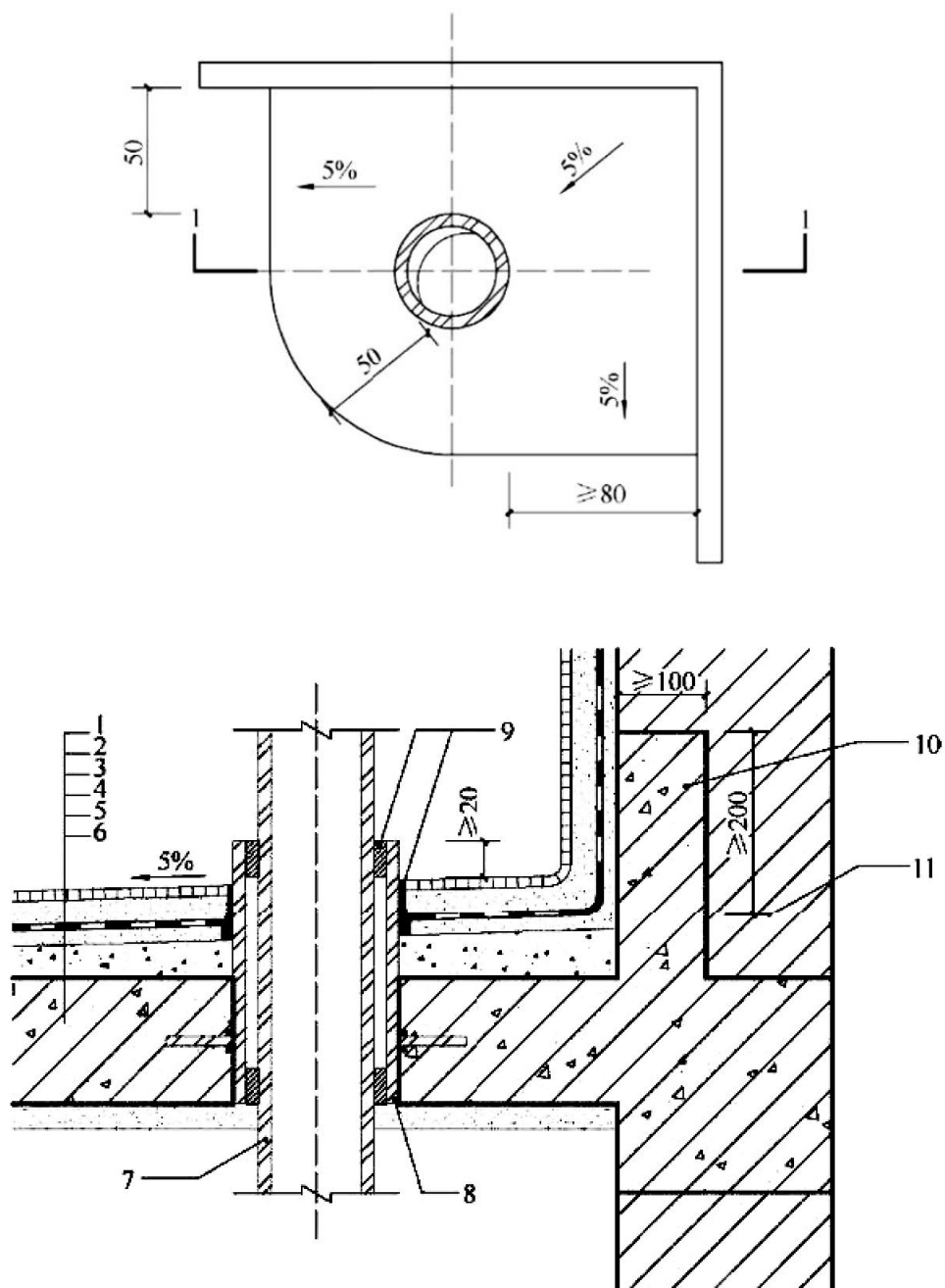
图 19.3.2-2 管道穿越楼板的防水构造
