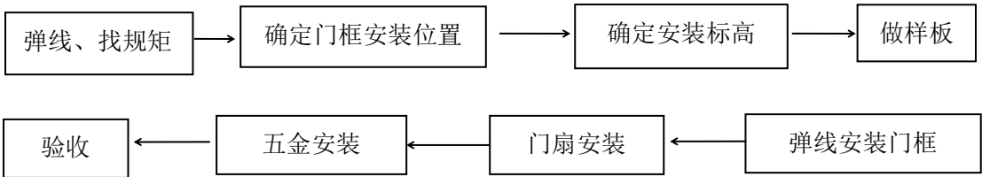
图 16.2.1 木门安装施工流程示意图
