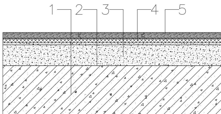
图 13.1.1 复合木地板安装构造示意图
