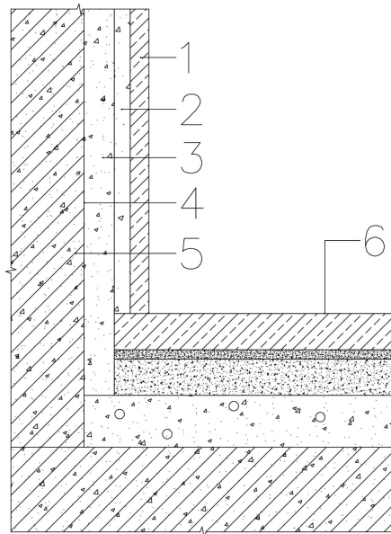
图 8.1.1 饰面砖粘贴构造示意图
