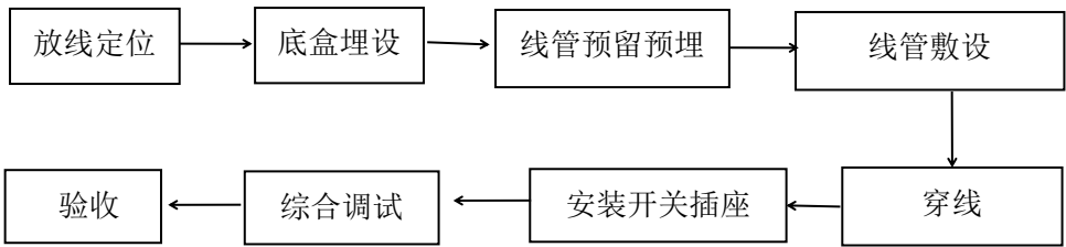
图 17.2.1 电气安装施工流程示意图
