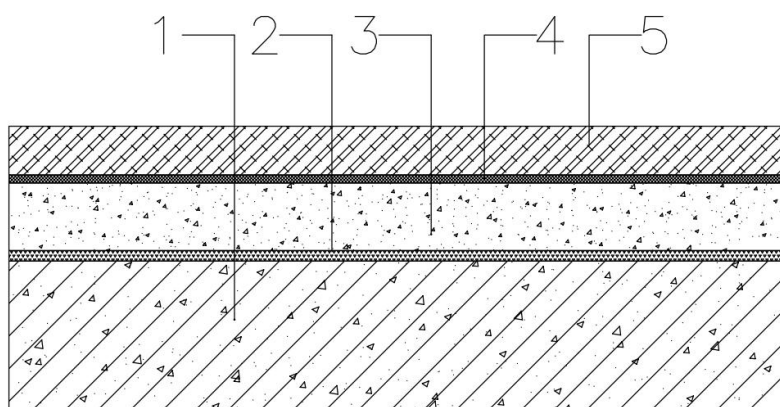
图 14.1.1 PVC 地胶安装构造示意图
