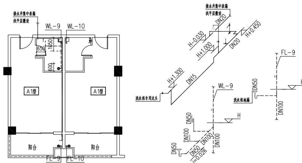
图 18.1.1 水电安装构造示意图
