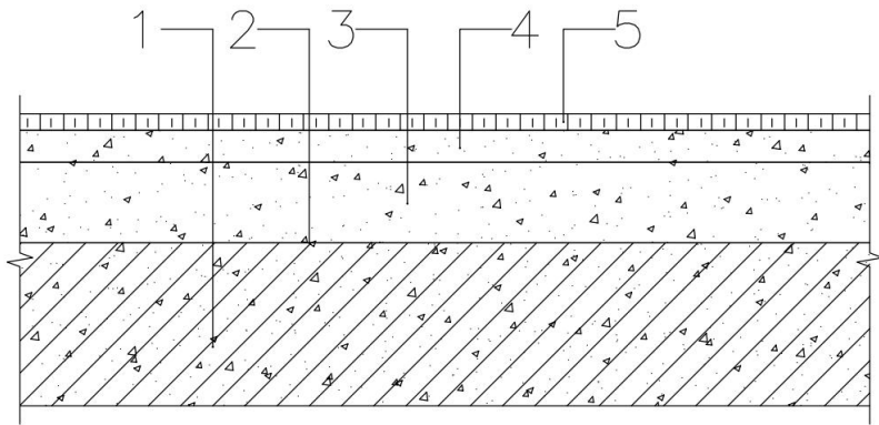
图 12.1.1 地面瓷砖铺贴构造示意图
