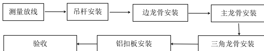
图 6.2.1 铝扣板吊顶施工流程示意图
