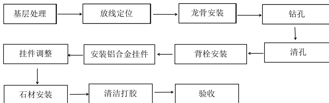
图 9.2.1 石材背栓式干挂施工流程示意图
