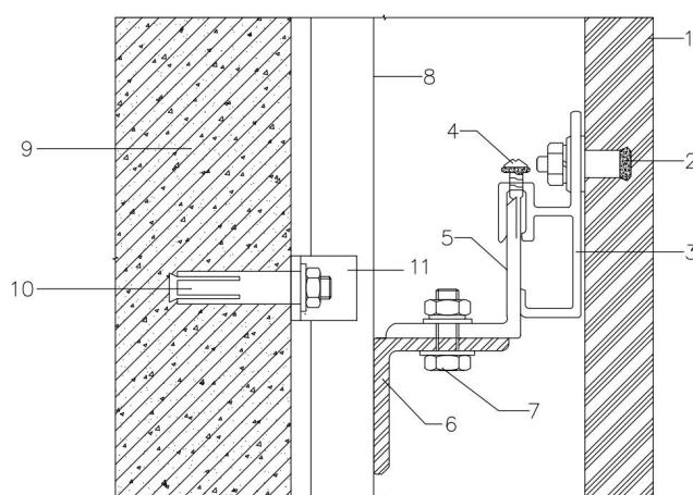
图 9.1.1 石材背栓式干挂构造示意图
